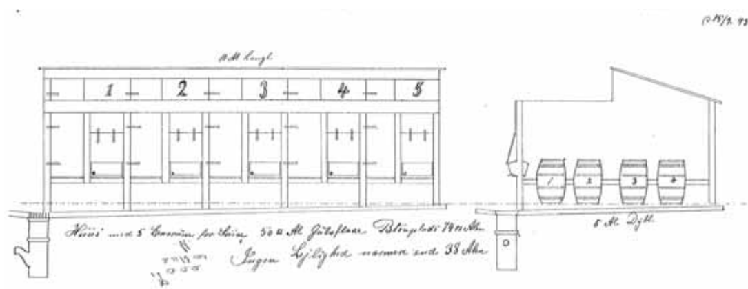
Tegningen af retiraden er dateret 1893, så det er ikke underligt at det i 1950-erne var i en sørgelig forfatning. Afstanden til lejlighederne skulle vær mindst 38 alen (knap 24 m). Tegning weblager.dk
