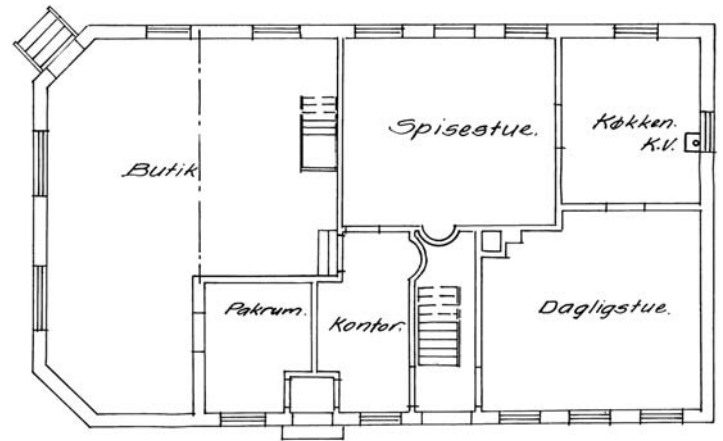
Plantagning over stueetagen efter udvidelse i Cathrinesminde. Tegning weblager.dk
